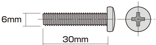
④ボルトM-A(M6×30mm)×4本
