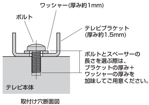
19 ボルトE (M8×25)
