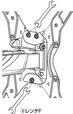
左右角度調節用ナット(上下3個)
