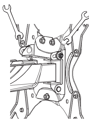
上下角度調節用ナット(左右2個)
