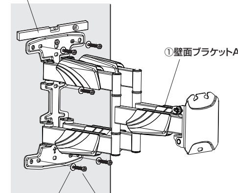
①壁面ブラケットA ⑩ワッシャーW-C ⑪ボルトW-A
