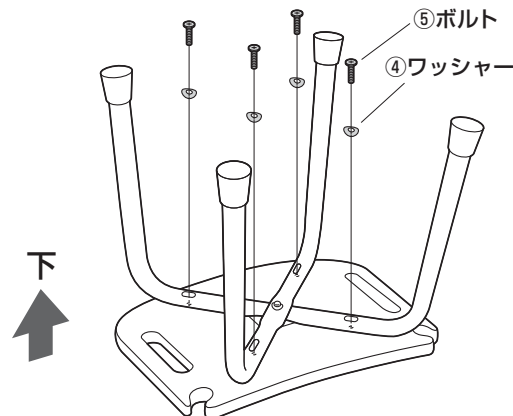
⑤ボルト [1/4"×38]
