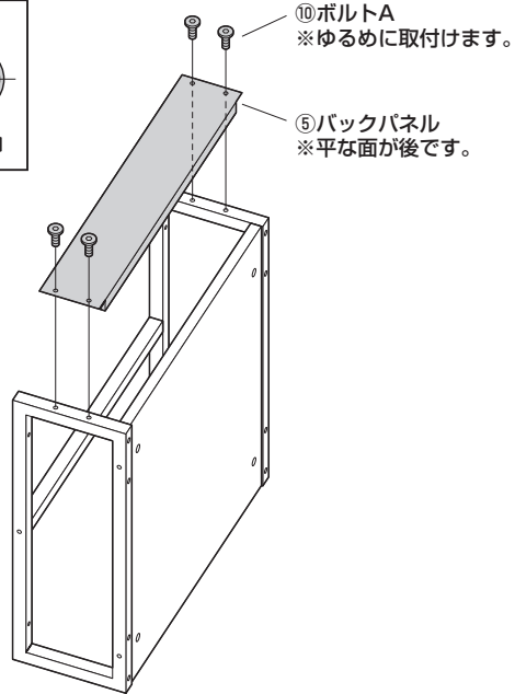
⑩ボルトA (M6×12)
