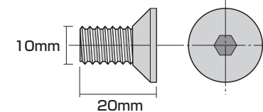
⑪ボルトK (M10×20mm) ×1本
