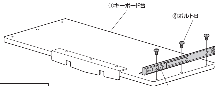
③右レール ※Rの表示があります。
