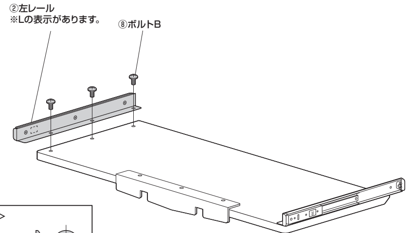
⑧ボルトB (M5×12mm)
