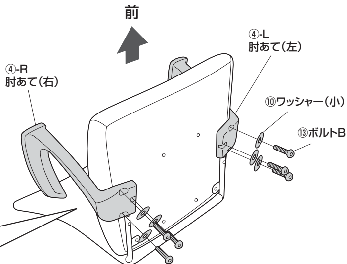
⑬ボルトB (M6×30)
