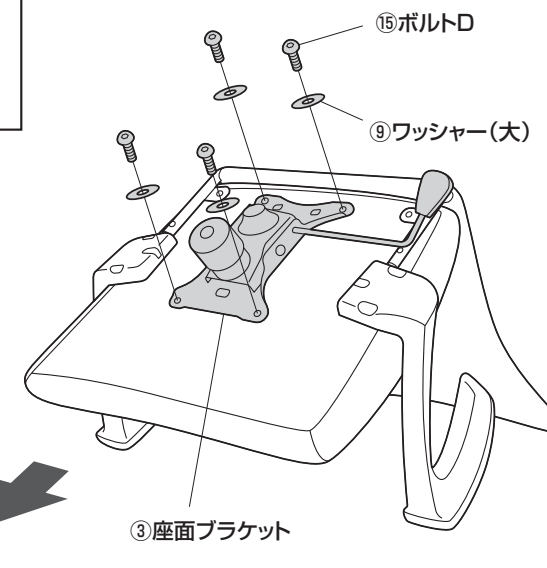
⑮ボルトD (M6×20)
