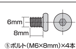
⑤ボルト（M6×8mm）×4本
